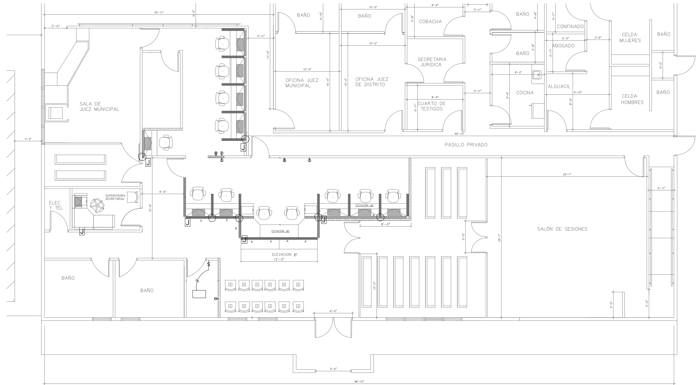
PLANO DE POWER POLE Y ELECTRICO ESCALA: 1/4" = 1'-0"
