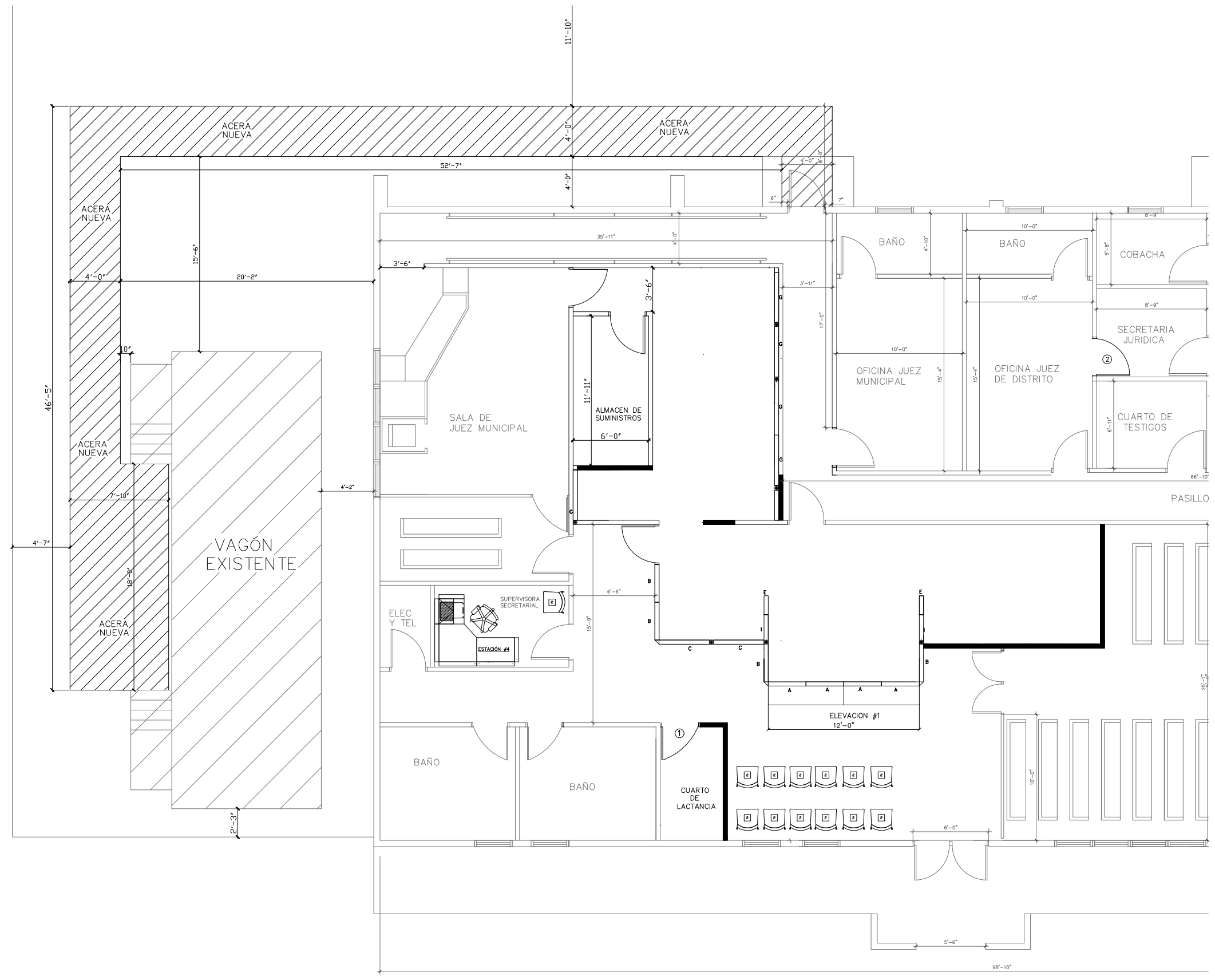
PLANO DE CONSTRUCCION ESCALA: 1/4" = 1'-0"
