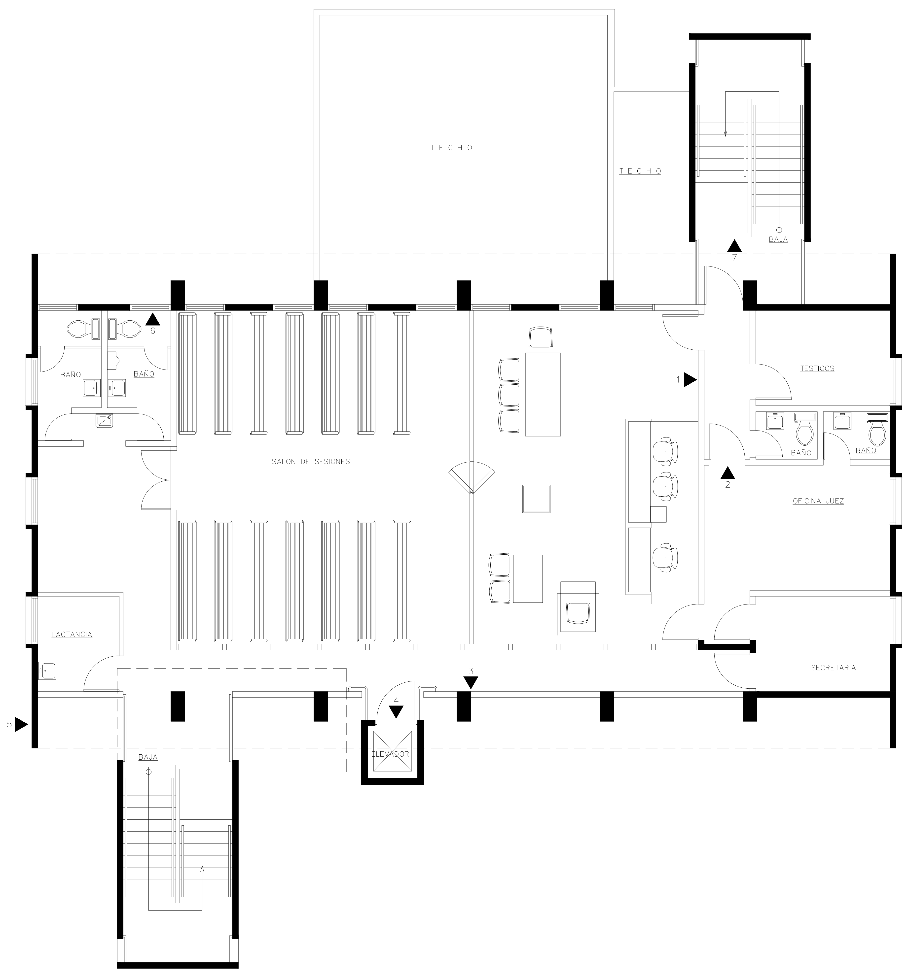
PLANO RESTAURACIÓN Y MEJORAS TPI CABO ROJO PISO 2 ESCALA: 1/4" = 1'-0"
